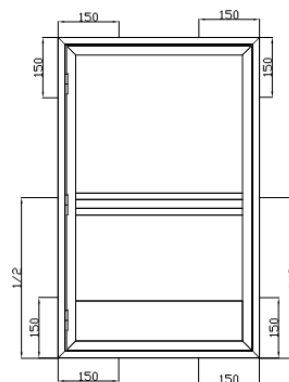
Montážní otvory pro jednokřídlé provedení
